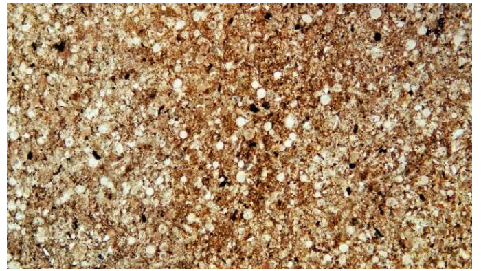
図 55 同左地点からの放散虫化石
