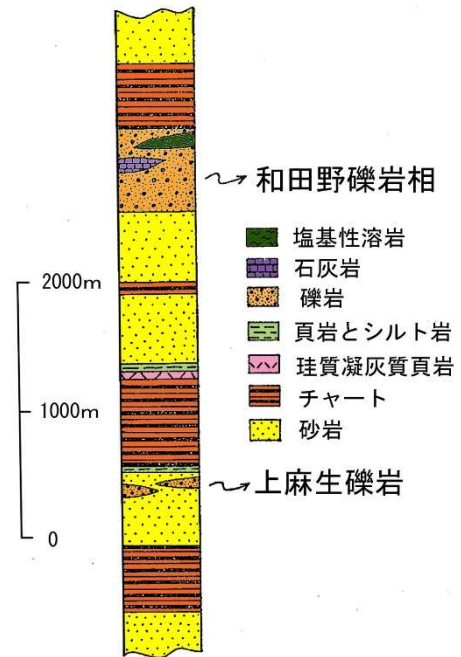
図 95 上麻生地域のペルム系柱状図
