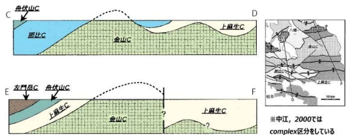
美濃帯の南北断面図（中江, 2000を改）
