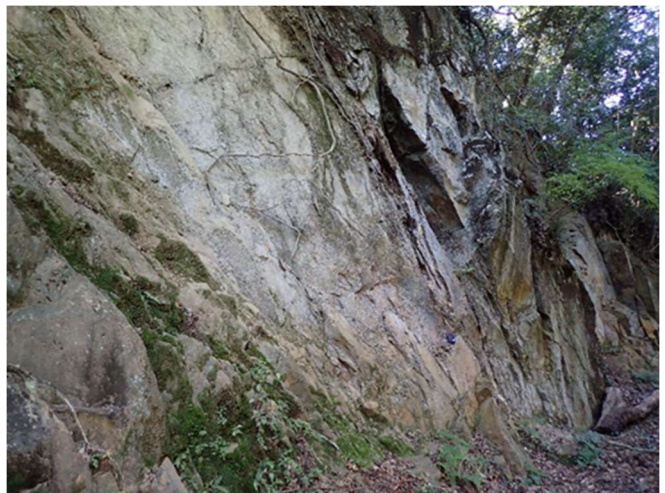
図 41 亀山市加太 不動の滝付近
