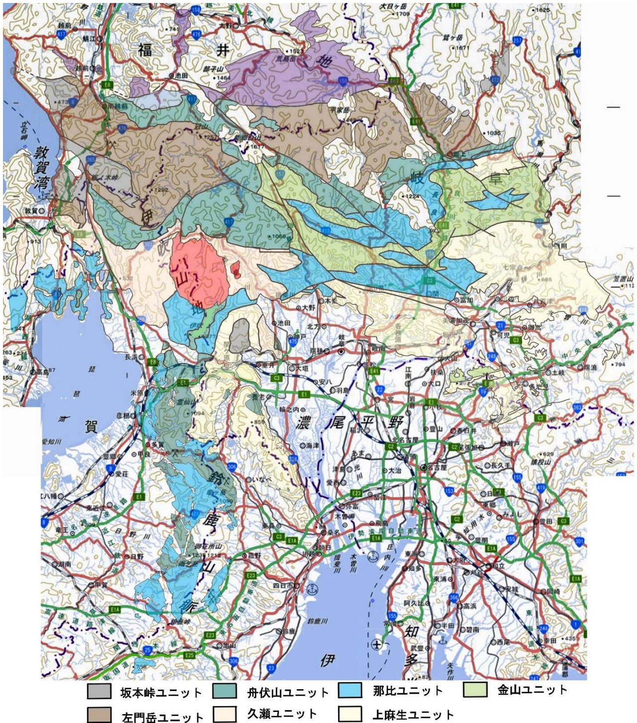
図5 美濃帯のユニット分布
