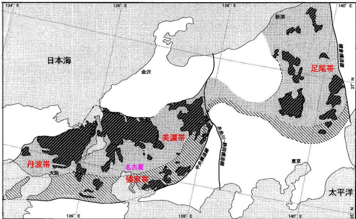
図1 美濃-丹波帯(太斜線の部分に露出している)
