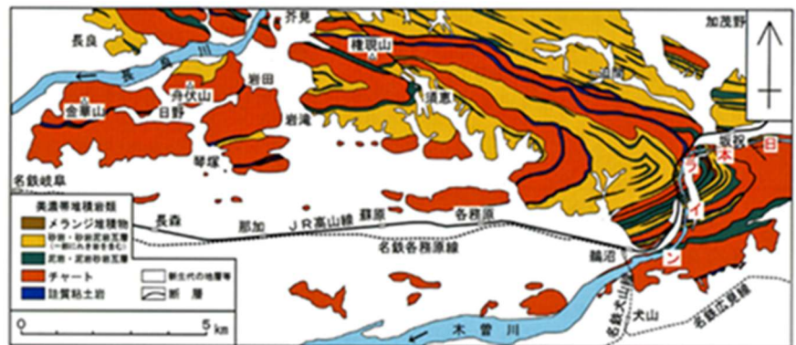
図 113 上麻生ユニットの組織地形 (小井土ほか, 2011)
