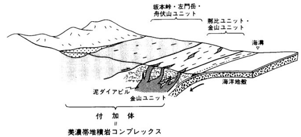
図 43 泥ダイアピルによる金山ユニットの貫入 (脇田, 1991)
