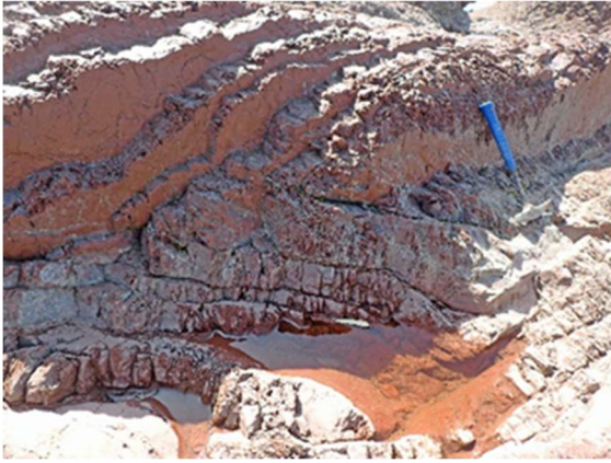
図 72 チャートの褶曲 鶯沼
