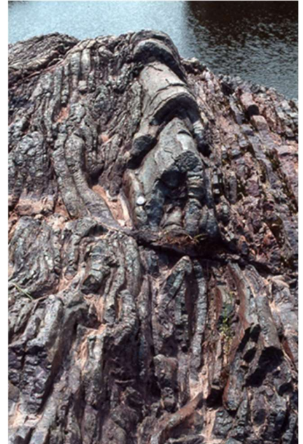
図 69 ポットホール 桃太郎園地北
