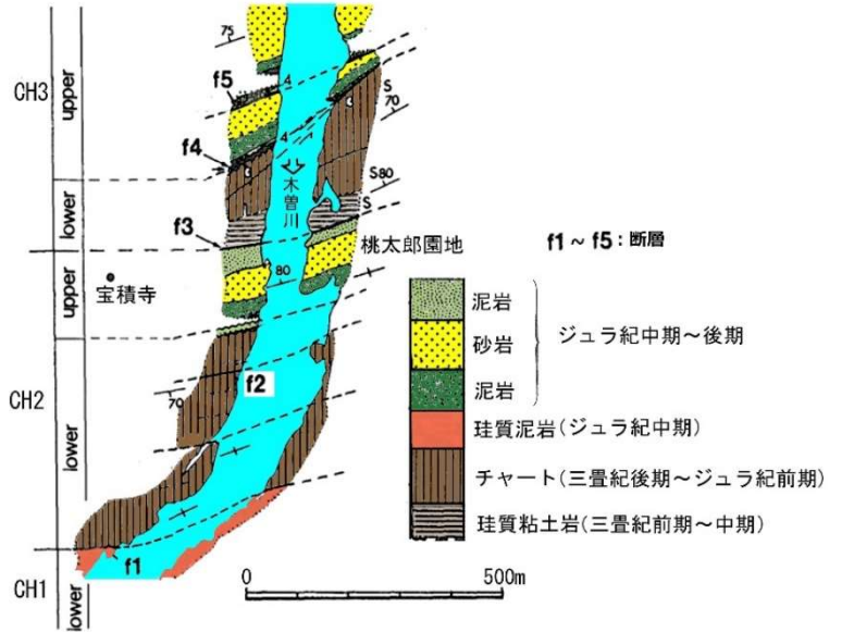
図 60 木曾川を挟んだ鵜沼-栗栖地域 Kimura, 1997 を改
